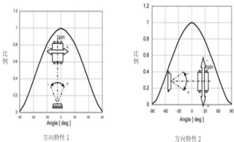
图 2.光照角度影响示意图
